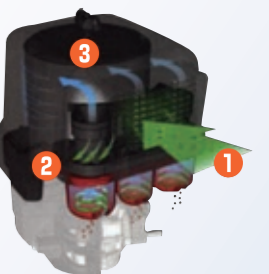
■サイクロンエアリーナ内部構造 ※イメージ図
