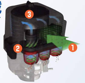
■サイクロンエアクリーナ内部構造 ※イメージ図
